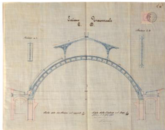
Sezione trasversale della tettoia in ferro, disegno allegato alla Perizia della Copertura in ferri e vetri della Galleria Vittorio Emanuele, 8 novembre 1868 (Milano, Archivio Storico Civico e Biblioteca Trivulziana, Piano Regolatore 1382)
